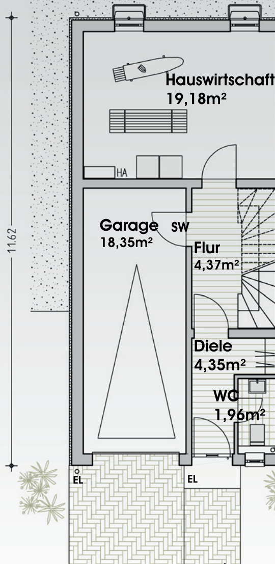
Haus 1 (Haus 7 gespiegelt)
